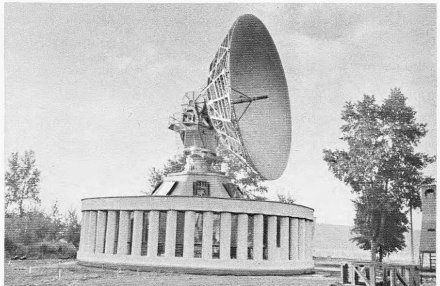
Bild 2. Eine der Standard-Bodenstationen für das russische System der Nachrichtensatelliten mit 12-m-Parabolspiegel. Diese Station steht im Gebiet Kemerowo zwischen Nowosibirsk und Krasnojarsk
