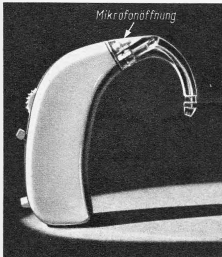
Links: Bild 8. Hinterdem-Ohr-Hörgerät (HdO). Die Mikrofonöffnung sitzt oberhalb des vom Hörer kommenden Schlauches (Robert Bosch Elektronik)
