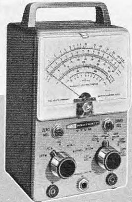
Universal- Röhrevoltmeter IM-18 D*
