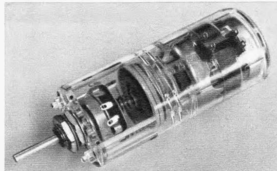
Bild 1. Ruwido-Motor-Drehwiderstand Typ 2002 für Fernbedienungen von Rundfunk- und Fernsehgeräten. Der Motor rechts treibt über ein Zahnradgetriebe und eine Rutschkupplung das Potentiometer links an
