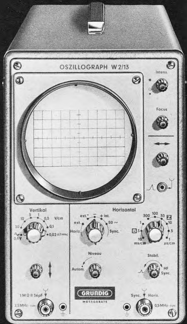
Werkstatt-Oszillograph W2/13
