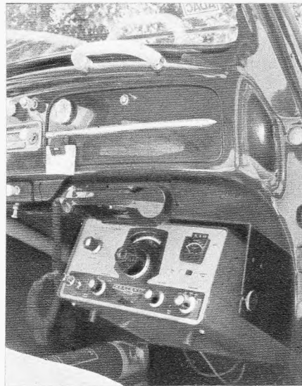
Bild 1. Bei dieser Einbauart bildet sich zwischen Transceiver und Armaturenbrett ein Warmluftpolster
