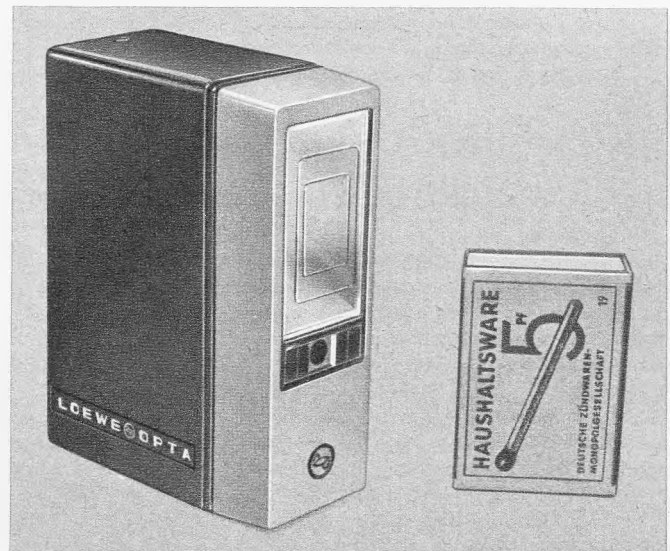
Rechts: Bild 2. Eine Leitzahl von 20 ist in diesem Blitzgerät untergebracht. Das Modell Loewe Optatron 420 C Computer gestattete diese Kompaktauweise u. a. durch Verwendung von Kleinleistungsthyristoren (Aufnahme: Dennewitz)
