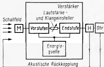
Bild 2. Grundsätzlicher Aufbau einer Hörhilfe [3]; M = Mikrofon, H = Hörer
