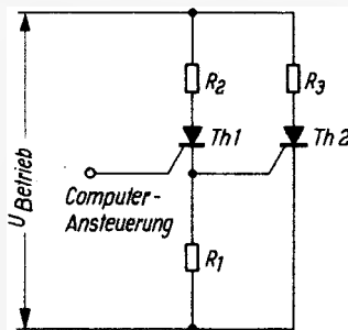
Bild 3. Prinzipschaltung einer beliebig erweiterbaren Thyristorkaskade
