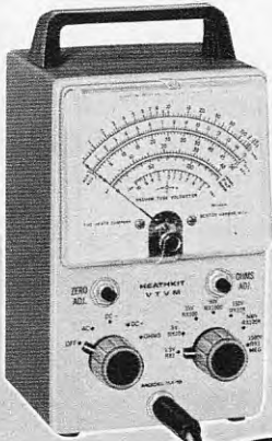
Universal- Röhrevoltmeter IM-18 E*
