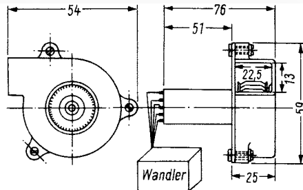
Bild 3. Die Abmessungen des Kleinstlüfters
