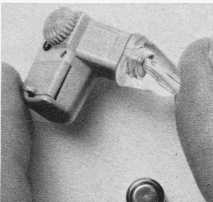
Bild 11. Im-Ohr-Hörgerät (IdO) von Philips für leichte bis mittlere Schwerhörigkeit. Das abschraubbare Ohrstück wird zweckmäßig individuell geformt und angepaßt, darunter die kleine Batteriezelle
