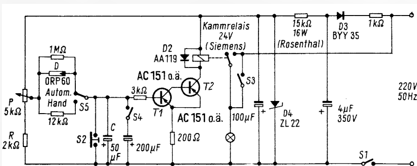
Schaltung des Belichtungsautomaten mit Transistoren
