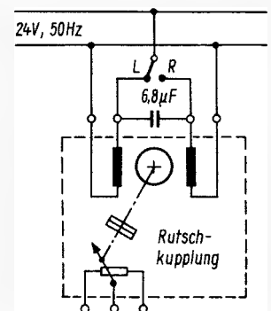
Bild 2. Schaltung des Motor-Drehwiderstandes für Rechts- und Linkslauf
